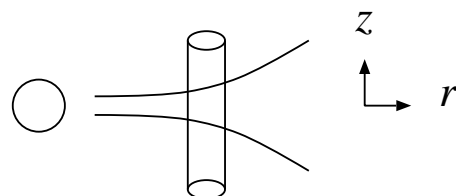
図 4.2: v_{in} > v_{out} 内側の粒子は外側の粒子に運動量を与える 内側の粒子はさらに内側へ
