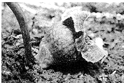
図1. 萼筒
