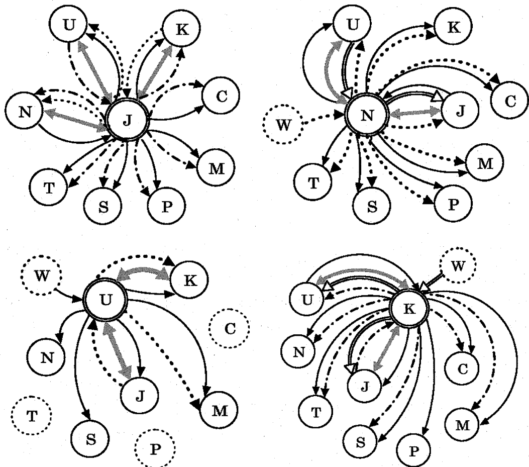
図6 Japan, Taiwan, Korea, U.S.A. 4カ国の上位 \overline{VS}_{pn \cdot km \cdot ql} の模式図
