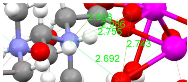
図 18 上) \text{Sr}_2[\text{EDTA-2H}]\text{Cl}_2 \cdot 5\text{H}_2\text{O} の分子内水素結合 ( d_{\text{N-O}} = 2.757 \text{ \AA}, 2.780 \text{ \AA} ) と分子間水素結合 ( d_{\text{N-O}} = 2.860 \text{ \AA} ) ; 下) \text{Sr}_2[\text{EDTA-2H}](\text{HCO}_3)_2 \cdot 4\text{H}_2\text{O} の分子内水素結合 ( d_{\text{N-O}} = 2.692 \text{ \AA}, 2.755 \text{ \AA} ) と分子間水素結合 ( d_{\text{N-O}} = 2.858 \text{ \AA}, 2.986 \text{ \AA}, d_{\text{O-O}} = 2.743 \text{ \AA} ) (Polyakova et al. 2009) [25].
