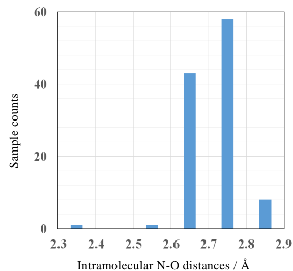
図 24 EDTA およびその塩における分子内窒素原子-酸素原子間距離の分布。
