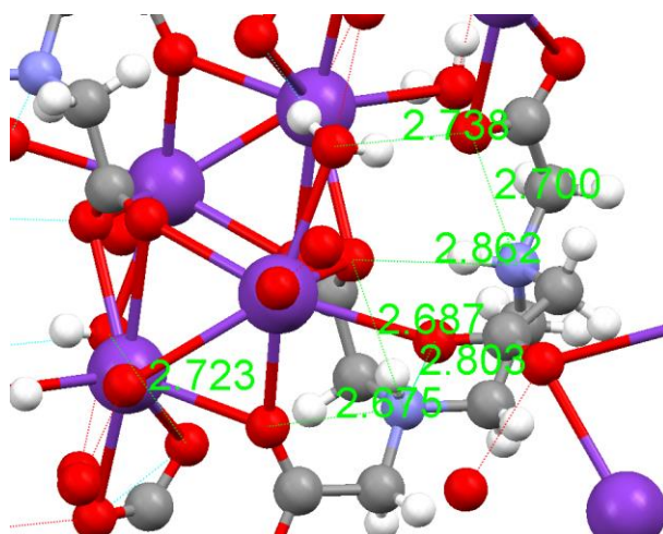
図 10 K 2 [EDTA-2H]·2H 2 O の分子内水素結合 ( d_{N-O} = 2.675 \text{ \AA} , 2.687 \text{ \AA} , 2.700 \text{ \AA} , 2.742 \text{ \AA} , 2.803 \text{ \AA} , 2.862 \text{ \AA} ) と分子間水素結合 ( d_{O-O} = 2.723 \text{ \AA} , 2.738 \text{ \AA} ) (Krawczyk & Lis 2011) [17].
