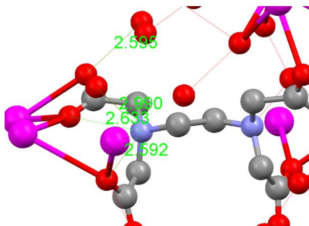
図 12 Rb 2 [EDTA-2H]·2H 2 O の分子内水素結合 ( d_{N-O} = 2.592 \text{ \AA} , 2.612 \text{ \AA} , 2.632 \text{ \AA} , 2.633 \text{ \AA} ) と分子間水素結合 ( d_{N-O} = 2.990 \text{ \AA} , d_{O-O} = 2.595 \text{ \AA} ) (Cotrait 1970) [19].
